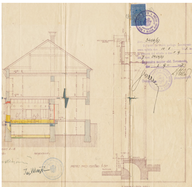
Prerez hiše z Mušičevim načrtom ureditve nove lekarnje in kleti na Rozmanovi ulici. 1937. Načrt hrani Andrej Mišo Andrijanič.
